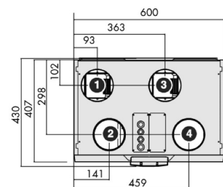
KN-KWL-96 SE-EC Draufsicht / Top view
