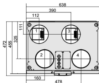
110 SE-EC Draufsicht / Top view
