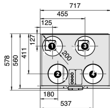
145 SE-EC Draufsicht / Top view
